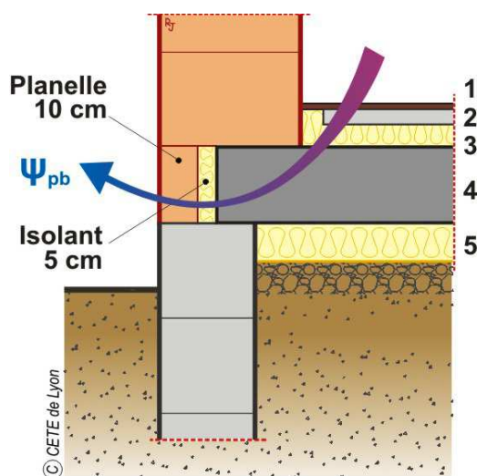
Traitement des ponts thermiques
